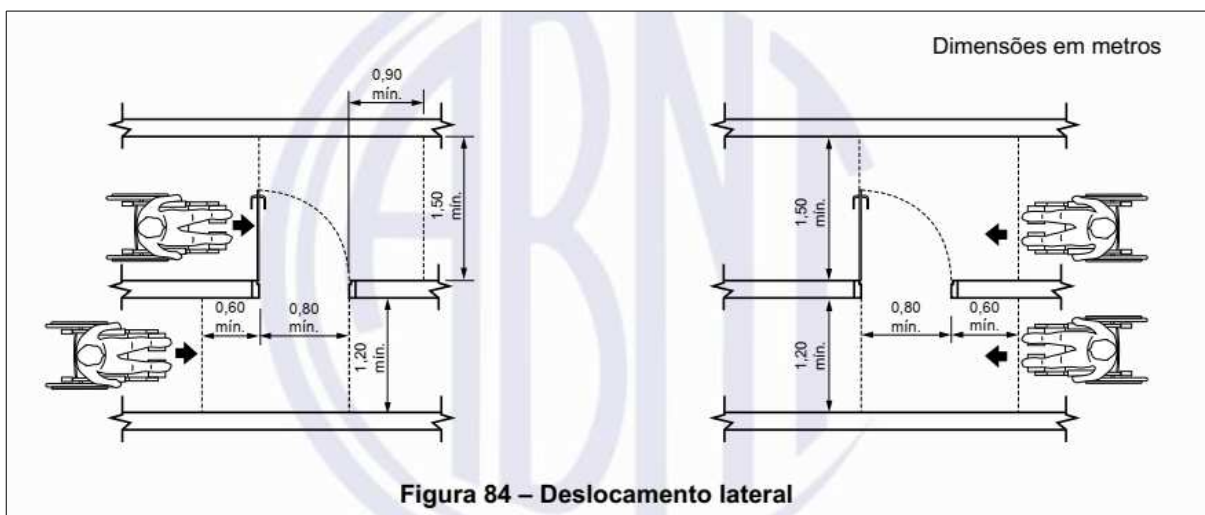
Figura 4: Figura 84, da NBR 9050:2020. Deslocamento lateral.
