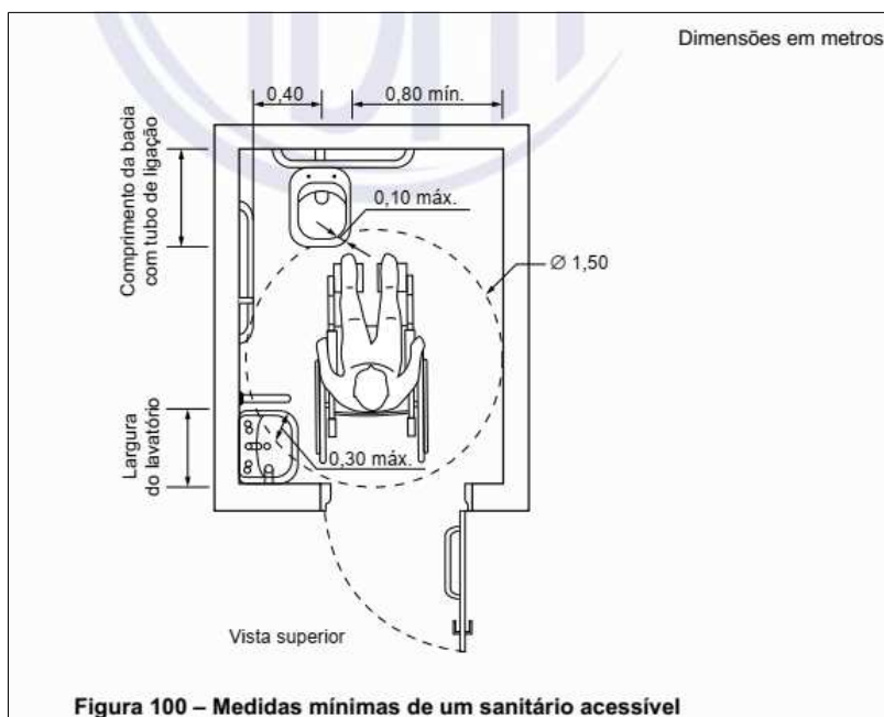
Figura 6: Figura 100, da NBR 9050:2020. Medidas mínimas de um sanitário acessível.
