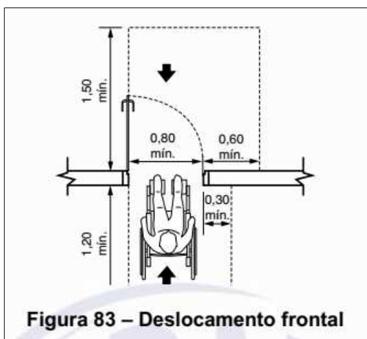
Figura 3: Figura 83, da NBR 9050:2020. Deslocamento frontal.
