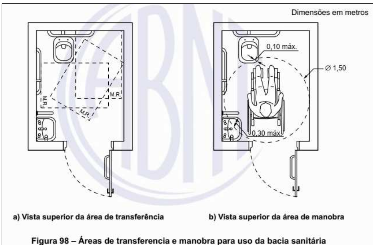
Figura 5: Figura 98, da NBR 9050:2020. Áreas de transferência e manobra para uso da bacia sanitária.
