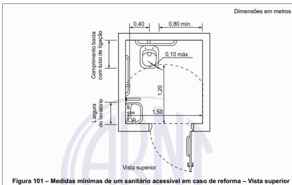
Figura 7: Figura 101, da NBR 9050:2020. Medidas mínimas de um sanitário acessível em caso de reforma.
